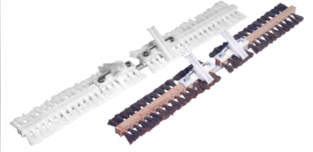
İrmik Sasör Fırçası Semolina Purifier Brush Щетка Ситовечной Машины
