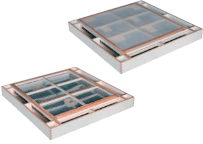
Elek Kasası Sieve Frame Рассевный Короб
